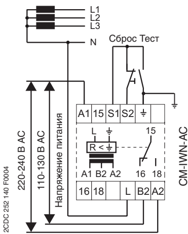
Трехфазная система IT-N
